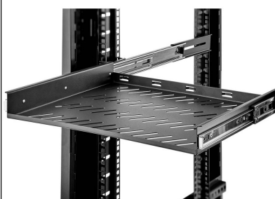
Étagère coulissante 1 U pour poser les équipements non - rackables
