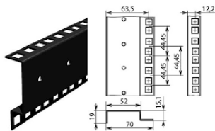
Doubles rails 19" à l'avant et à l'arrière
