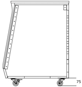
4 Roulettes haute résistance dont 2 avec freins - apparentes
