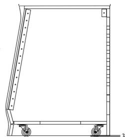
4 Roulettes haute résistance non apparentes
